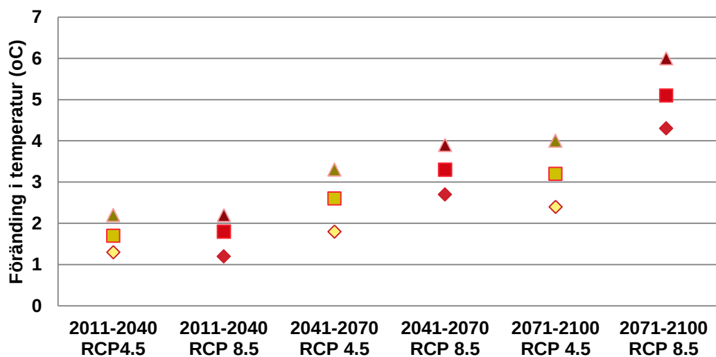
Figur 8. Osäkerheter i scenarier av temperaturförändringar beroende på val av emissionsscenarie och vilken modell som använts. För respektive tidsperiod och val av RCP (gul = RCP4.5 och röd=RCP8.5) visas högsta (triangel), medel (kub) och lägsta modellberäknade temperaturförändring (romb) jämfört med 1961-1990 35 .
